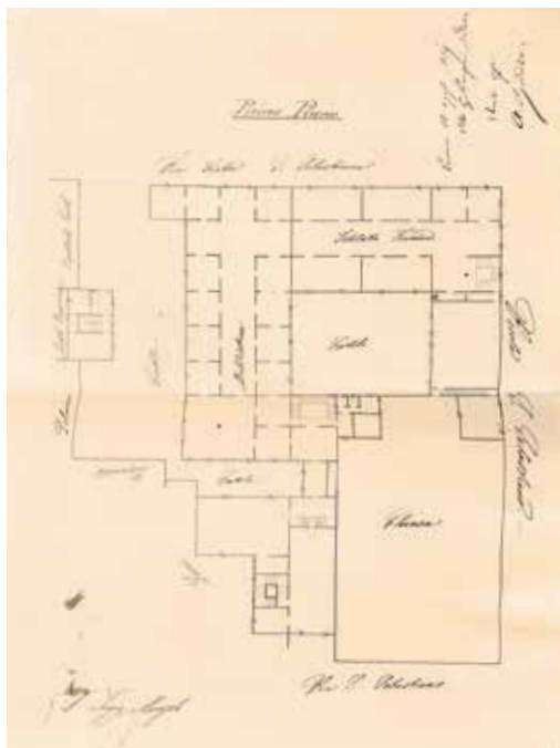
Fig. 28 a, b, c. Planimetrie dei locali destinati all'Istituto industriale e professionale di Verona presso l'ex Collegio di San Sebastiano, 1869 (ASVr, Comune di Verona - parte moderna, Consuntivi , b. 46, ex I-II-9, Spese d'amministrazione , pratica 10 agosto 1869).
