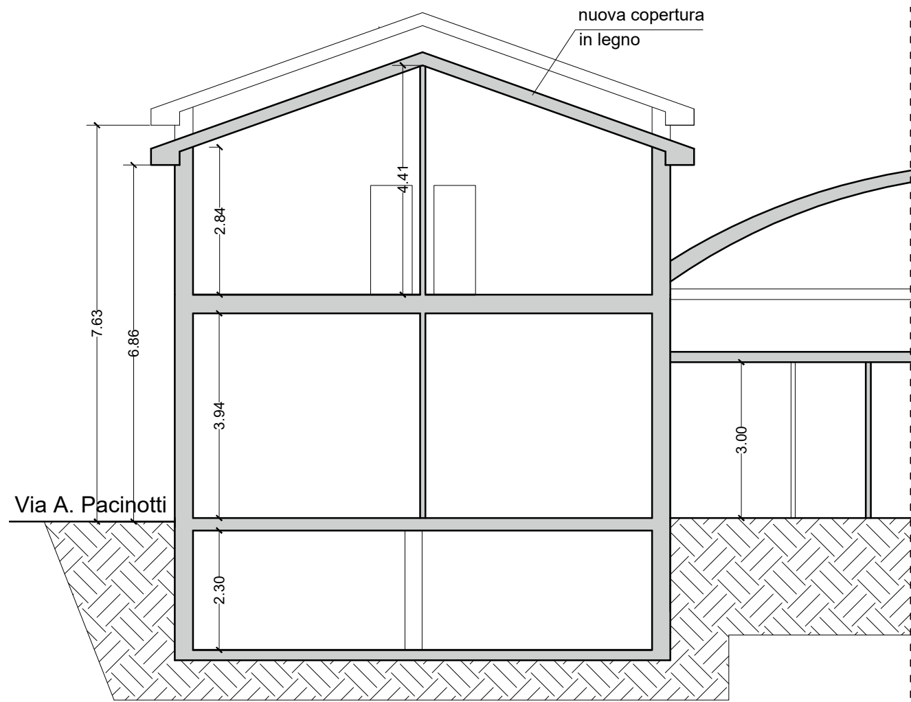
SEZIONE D - D SCALA 1:100
